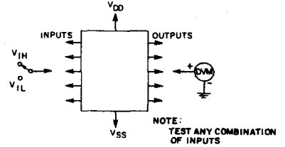
Fig. 16 - Input voltage.
