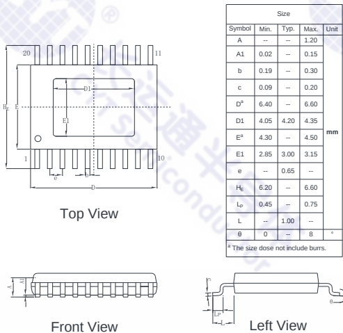
TSSOP20
