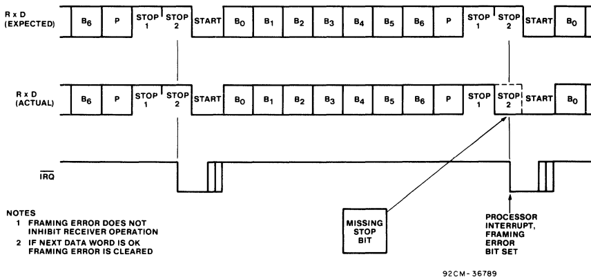
Fig. 15 - Framing error.
