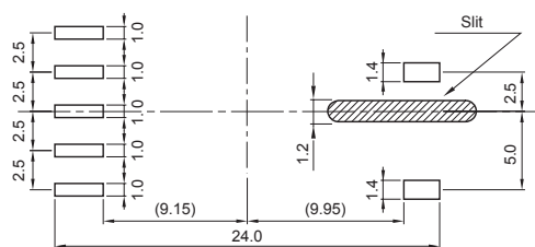
LAND PATTERNS (mm) 推奨ランド寸法
