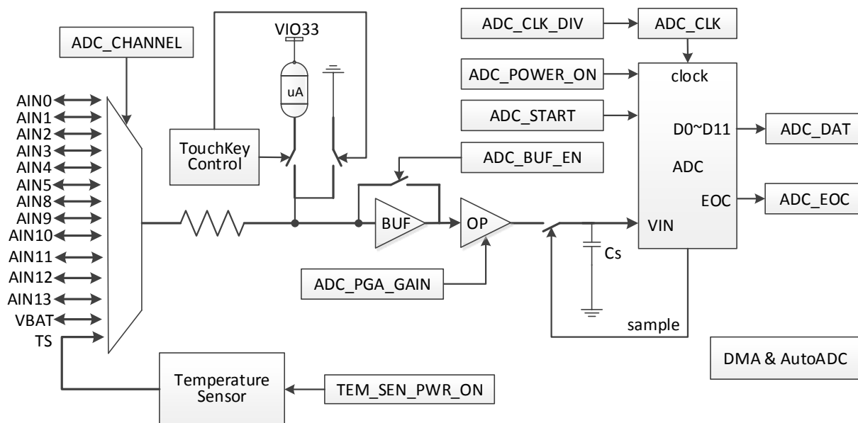
图 15-1 ADC 结构图
