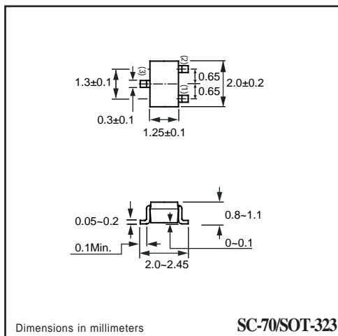
SC-70/SOT-323
