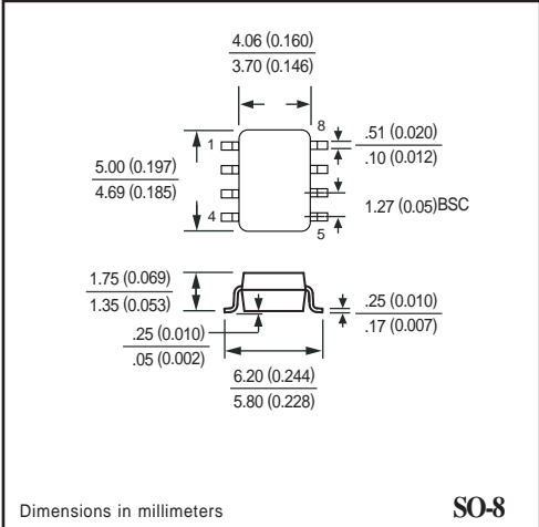
SO-8
