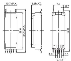
DIMENSIONS (mm) 外形寸法図
