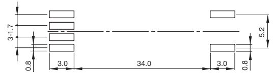
LAND PATTERNS (mm) 推奨ランド寸法
