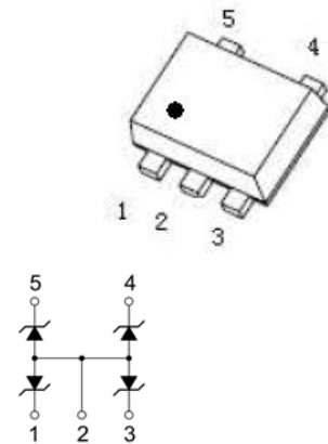
SOT-553
