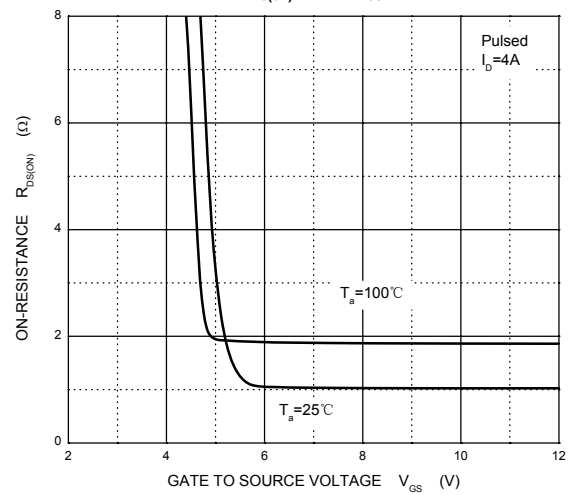
R_{DS(ON)} — V_{GS}
