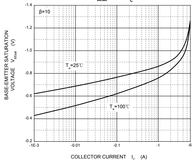
V_{BEsat} — I_c
