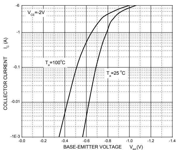
I_c — V_{BE}
