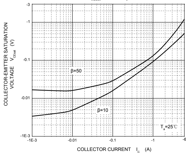
V_{CEsat} — I_c
