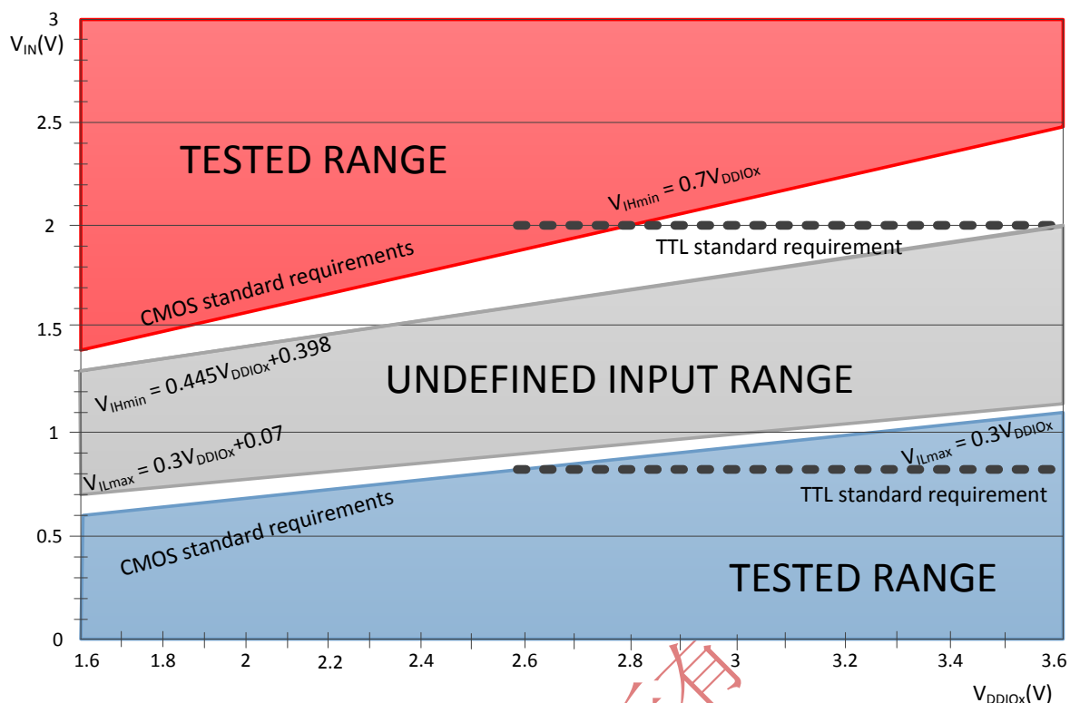
图 17 TC 和 TTa 的 I/O 口输入特性
