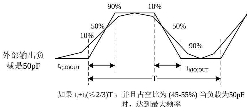
图 19 输入输出交流特性定义
