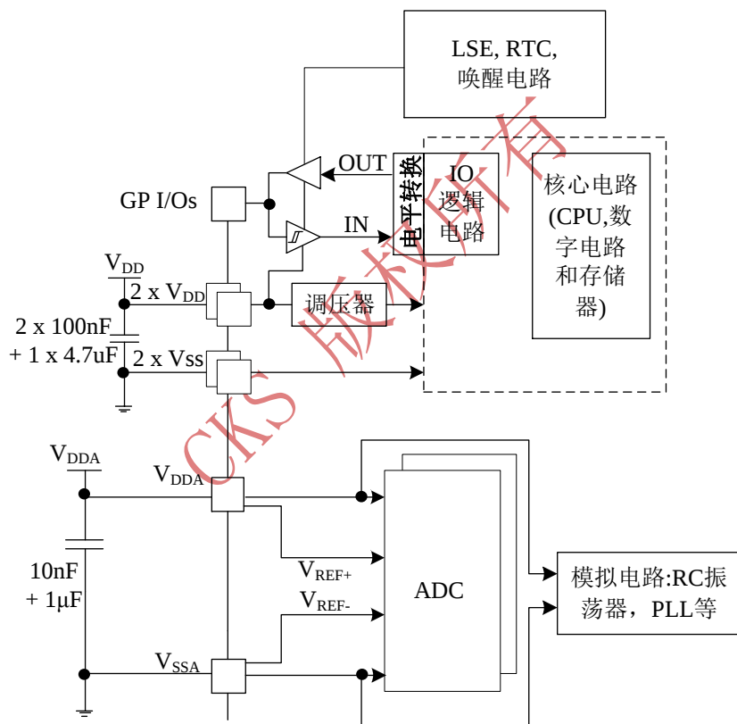
图 11 供电方案
