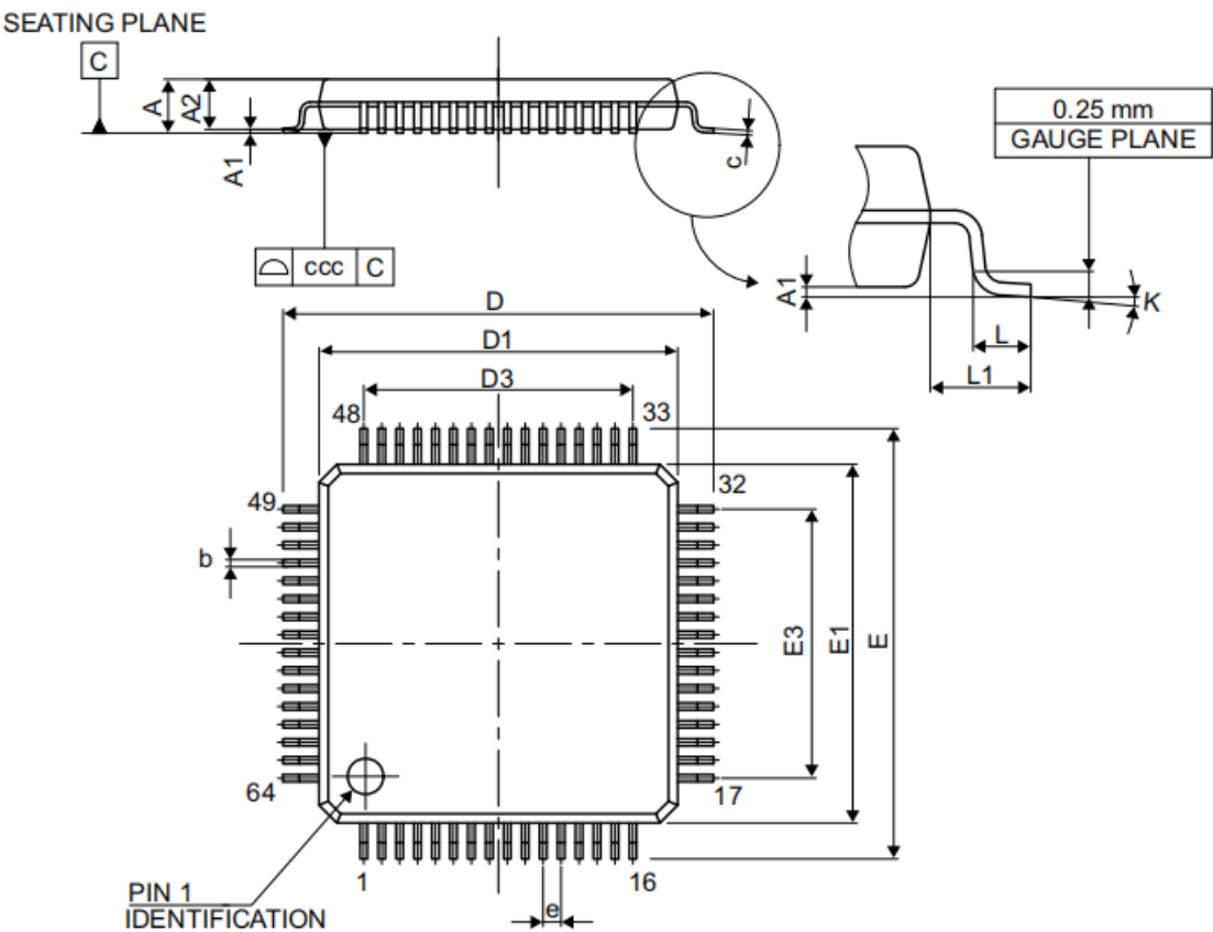
图 54 LQFP64，64 脚底剖面方形扁平封装图
