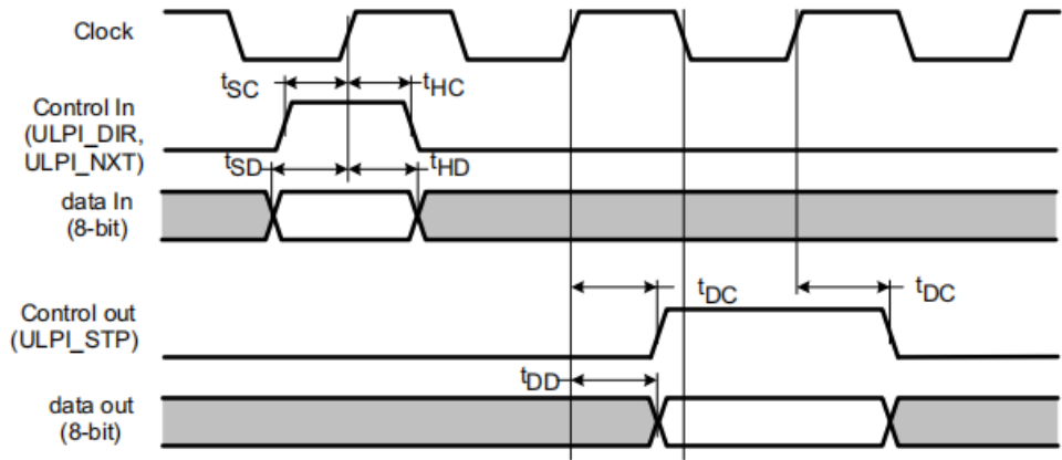
图 24 ULPI 时序图
