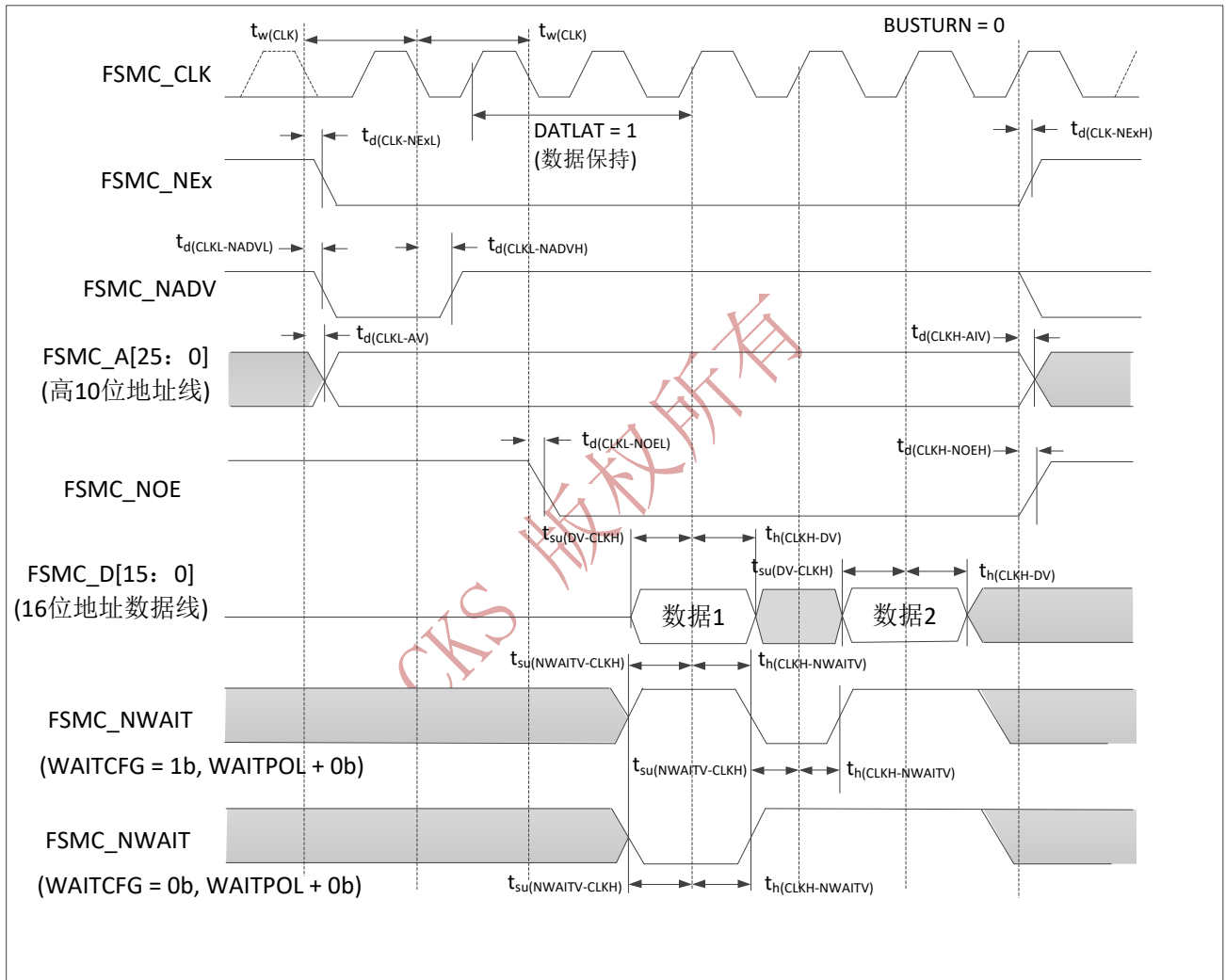
图 39 同步非总线复用 NOR/PSRAM 读时序
