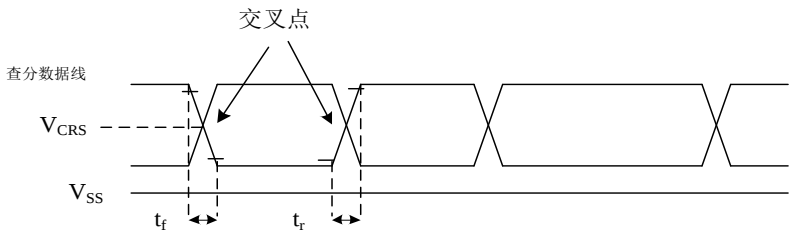
图 23 USB 时序：数据信号上升和下降时间定义
