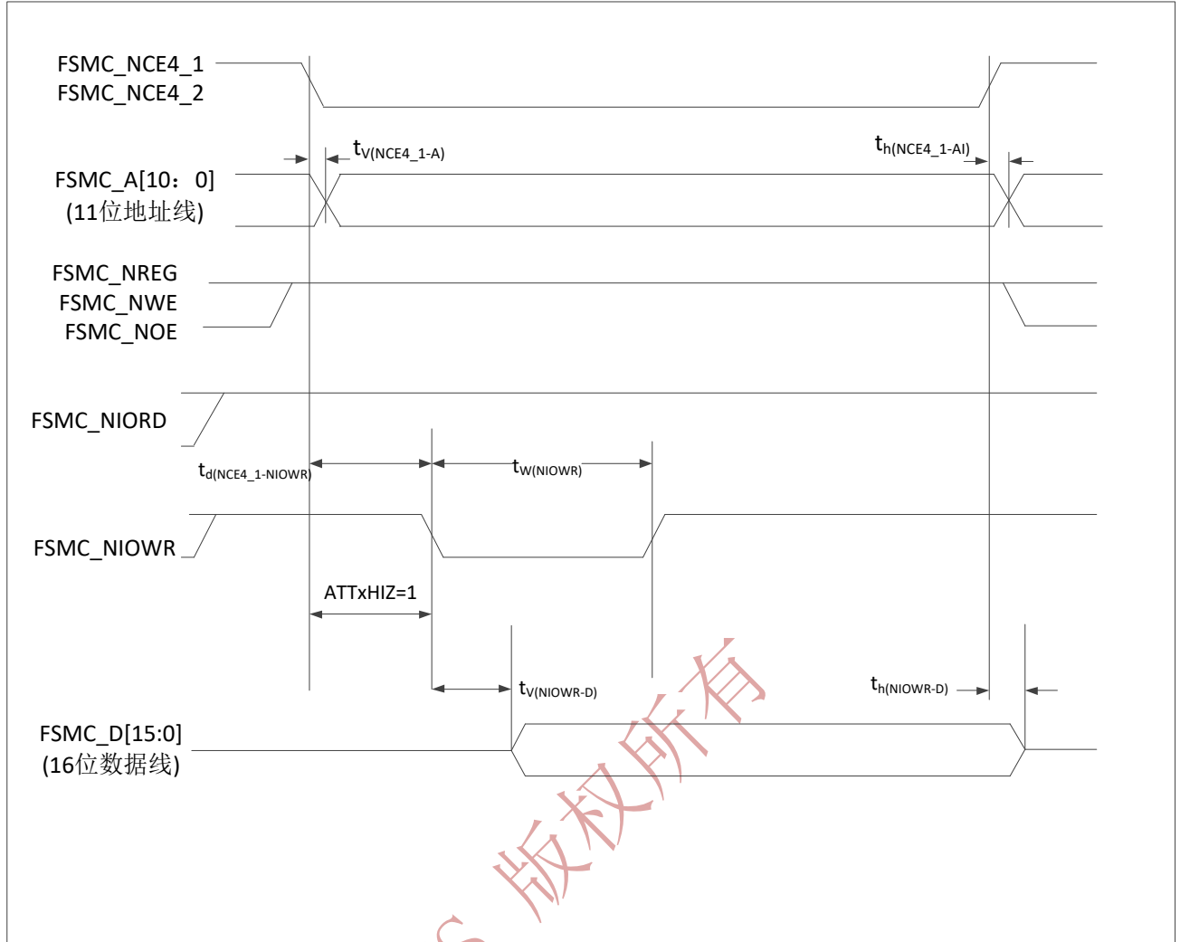
图 46 I/O 空间写操作的 PC 卡/CF 卡控制器波形
