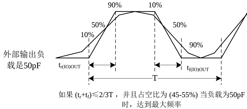
图 16 输入输出交流特性定义
