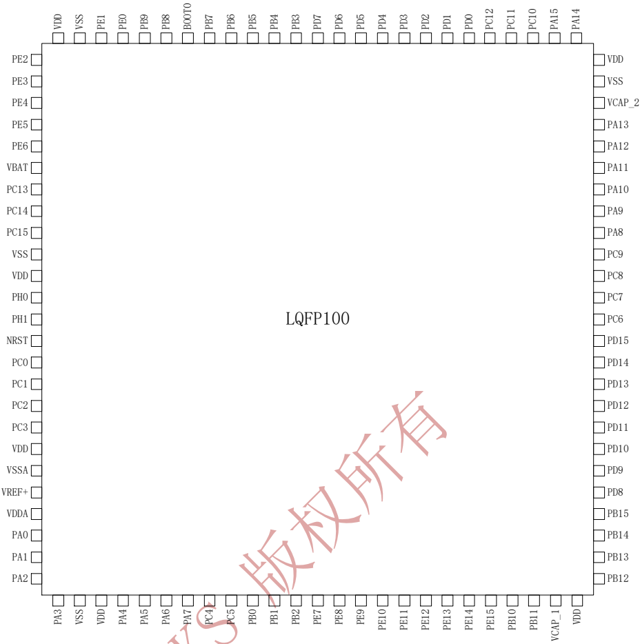
图 5 LQFP100 引脚分布
