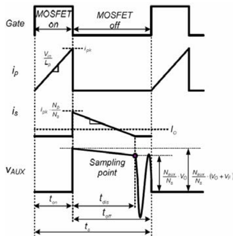
图2 辅助边电压波形
