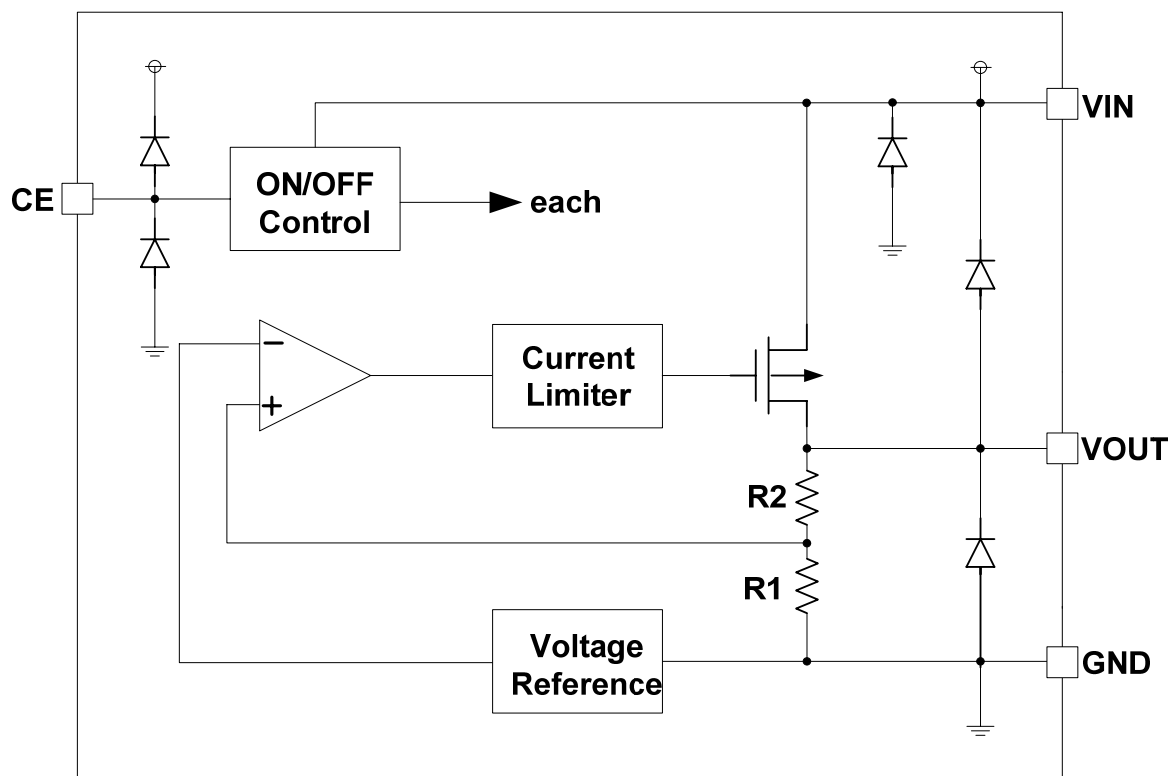
功能块框图
