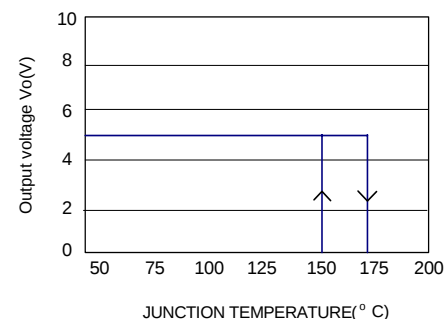
Thermal protection
