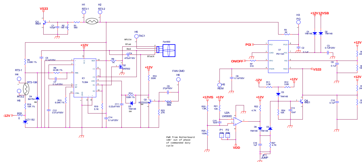
Fan Protection
