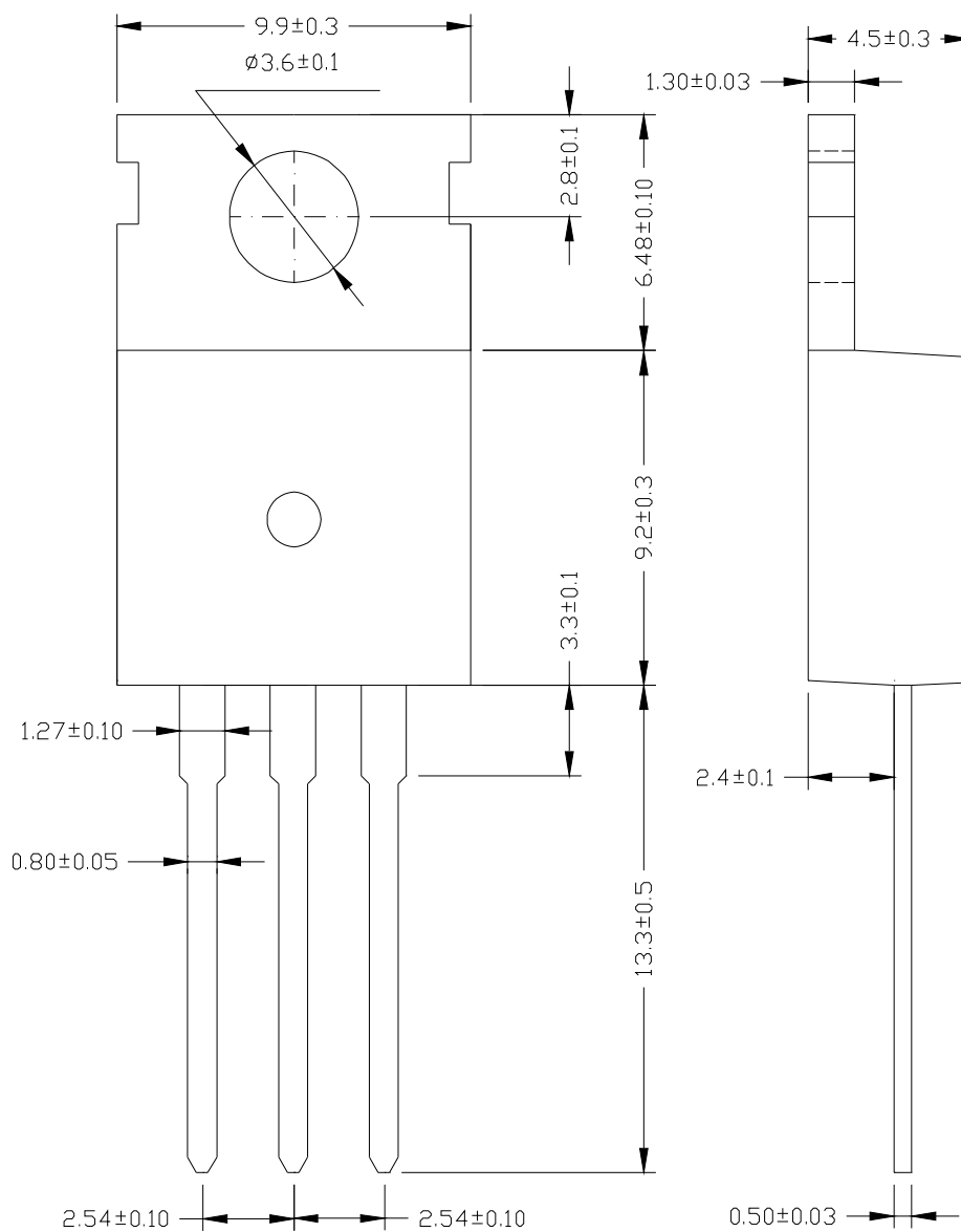
TO-220A
