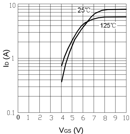
图 3 传输特性曲线
