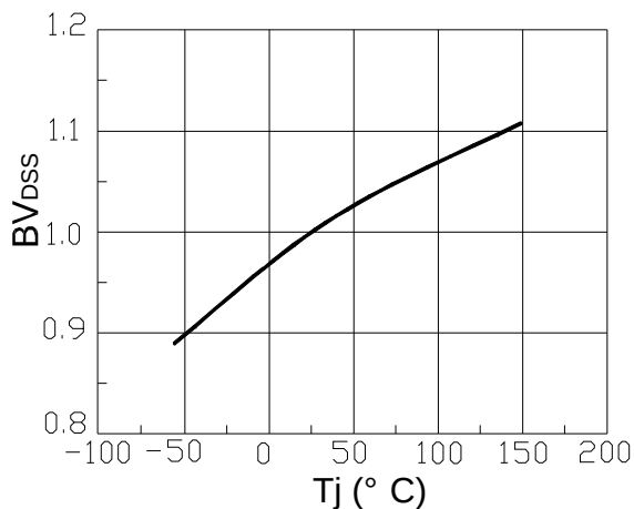
图 5 击穿电压-温度关系曲线
