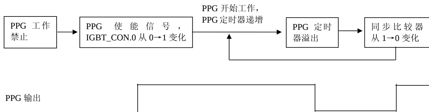
图 12.1.1 PPG 输出时序控制
