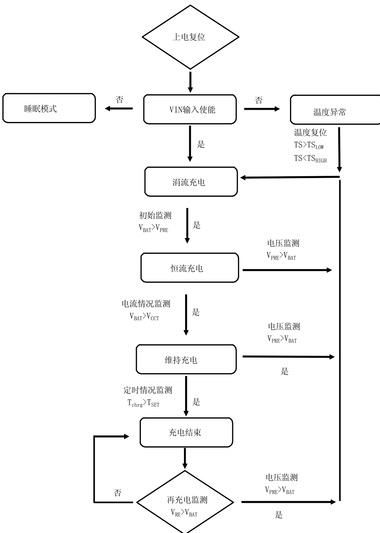
图3 充电工作框图
