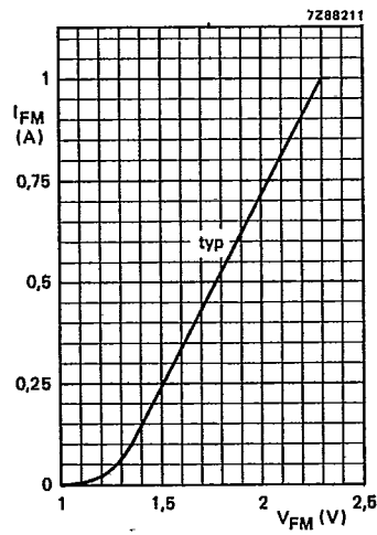
Fig. 6 T_{amb} = 25\text{ }^{\circ}\text{C} ; t_p = 10\text{ }\mu\text{s} ; \delta = 0.01 .
