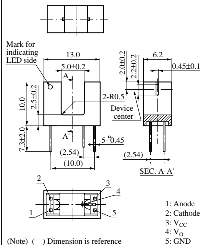
CNZ1403A/B
