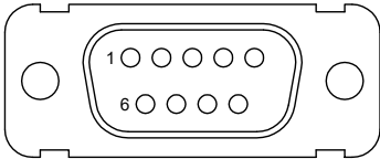
“-S OPTION” 9-PIN D-SUB CONNECTOR (Example: CCR-33S10-S)
