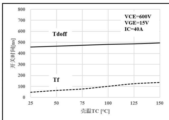
图 11 关断温度特性
