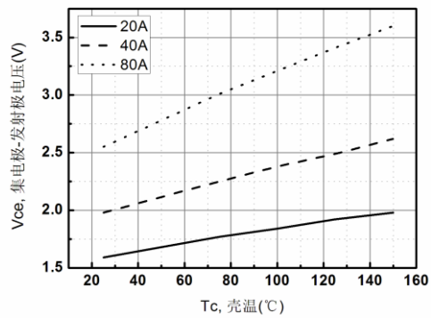
图 4 饱和压降温度特性(Vge=15V)
