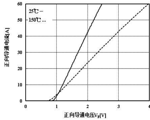
图 16 二极管正向特性
