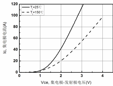
图 3 饱和压降特性(Vge=15V)
