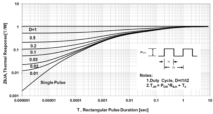
图 18 瞬态热阻特性
