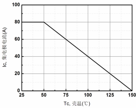
图 15 集电极电流温度特性
