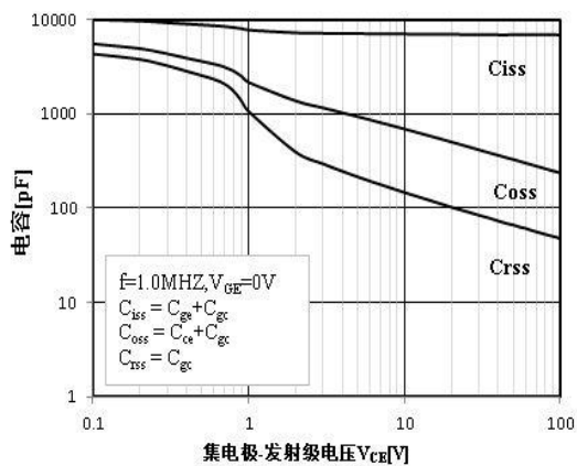
图 5 电容特性
