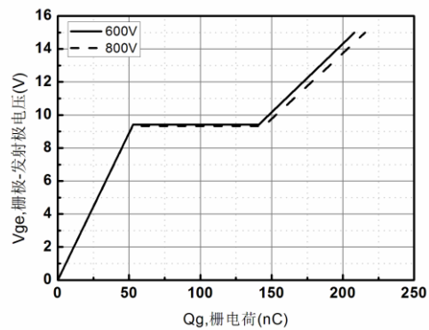
图 6 栅电荷特性
