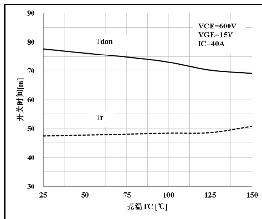
图 10 开通的温度特性
