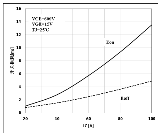
图 12 开关损耗的电流特性
