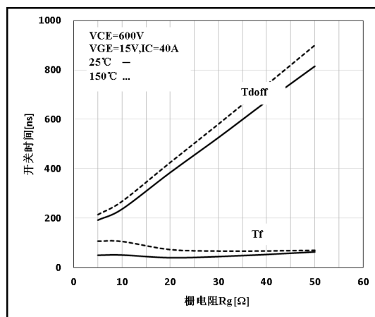
图 8 关断-栅电阻特性曲线
