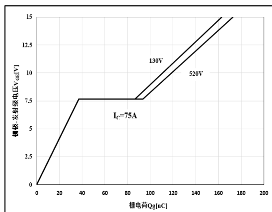
图 18 栅电荷特性
