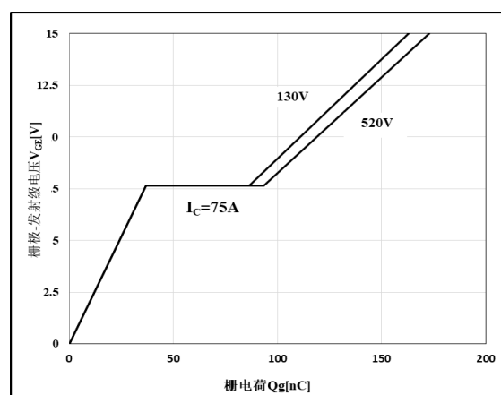
图 18 栅电荷特性
