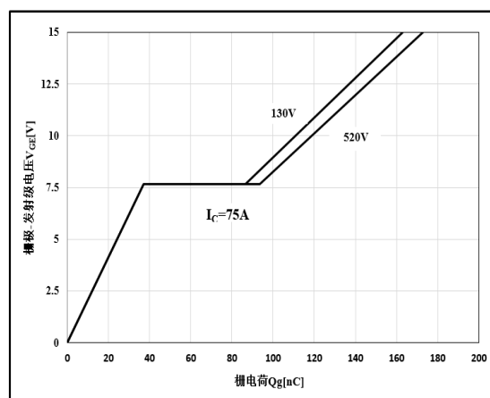
图 18 栅电荷特性
