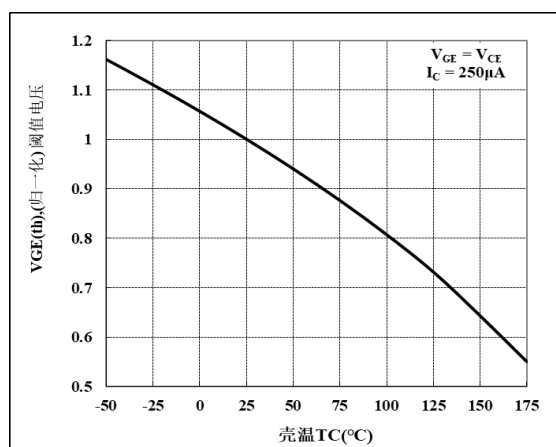
图 20 阈值电压温度特性
