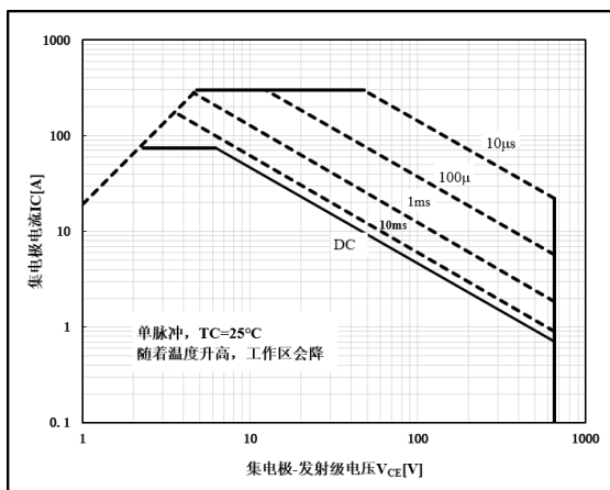
图 21 正向安全工作区
