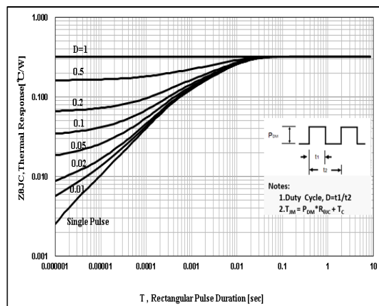
图 22 瞬态热阻特性
