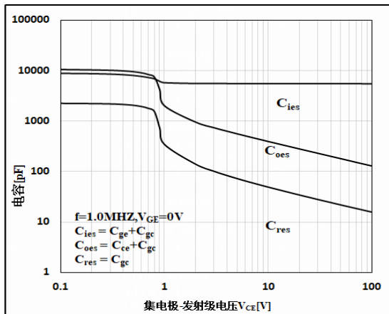
图 5 电容特性
