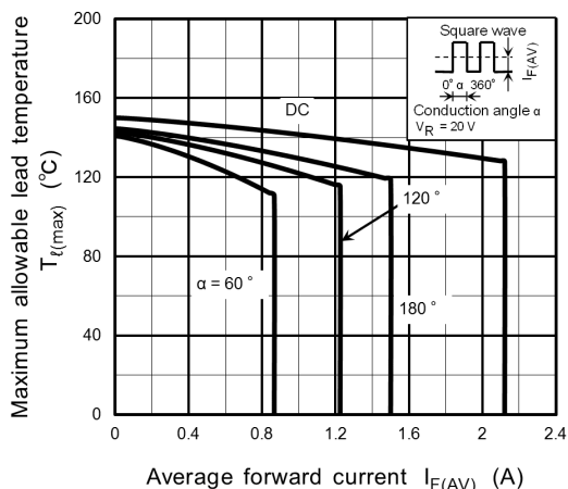
Fig. 10.4 T_{t(max)} - I_{F(AV)}
