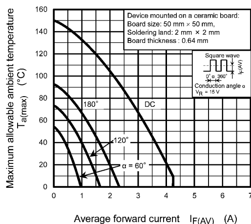
Fig. 10.3 T_{a(max)} - I_{F(AV)}
