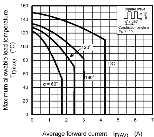
Fig. 10.4 T_{l(max)} - I_{F(AV)}
