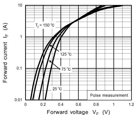
Fig. 10.1 I_F - V_F
