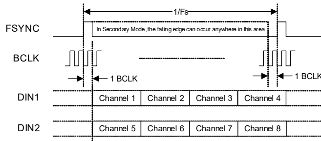
Figure 4-15. TDM Data Format—2 x DIN
