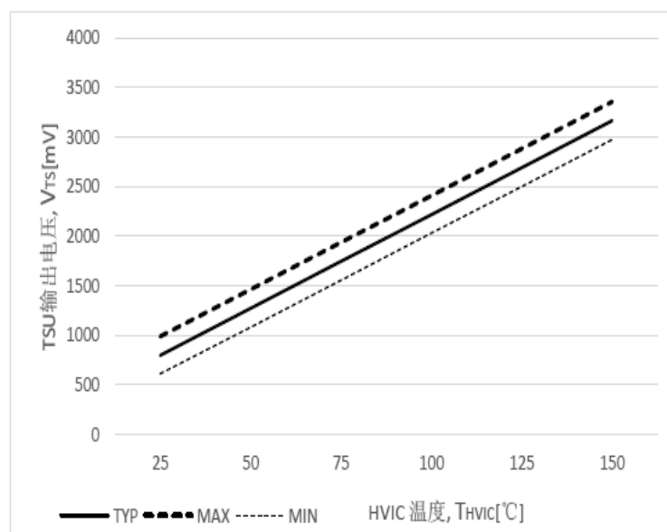
V_{TS} 电压的温度特性
