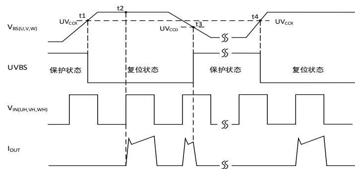
欠压保护（高侧）
