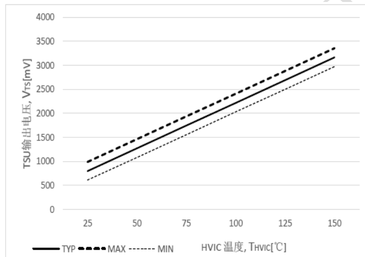
V_{TS} 电压的温度特性
