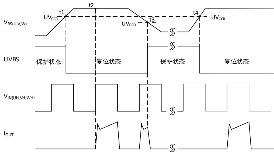
欠压保护（高侧）
