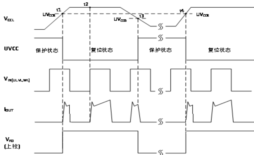
欠压保护（低侧）
