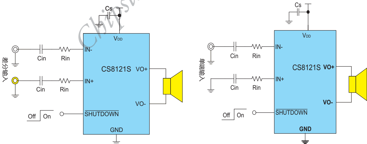
图2 CS8121S单端输入方式应用图
