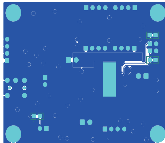
DEMO BOARD 底层图
