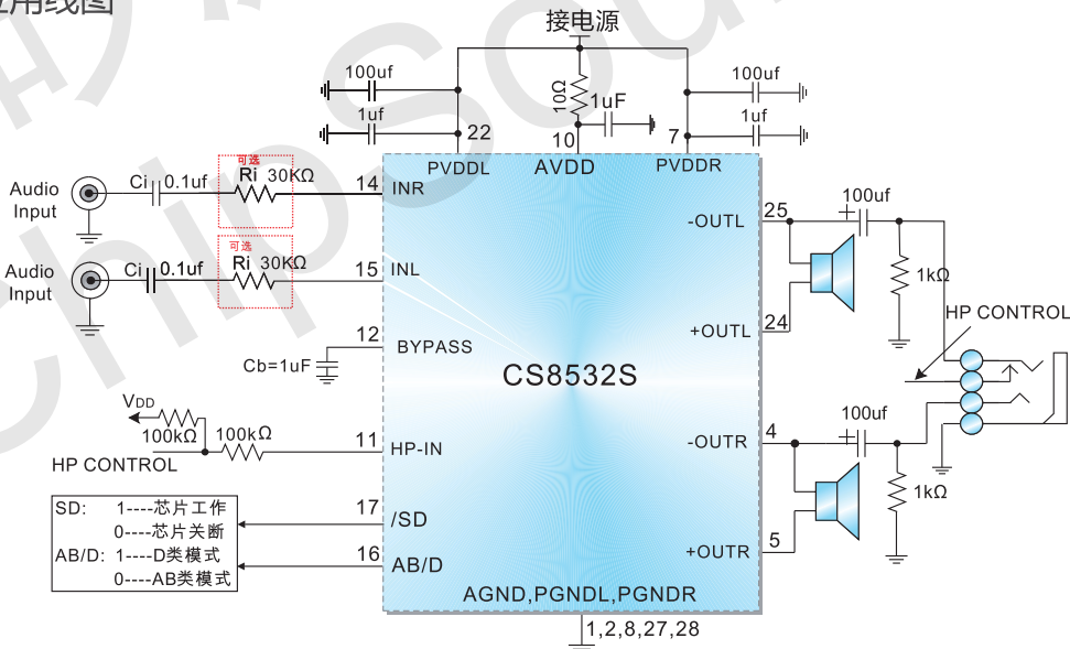
CS8532S应用电路图
