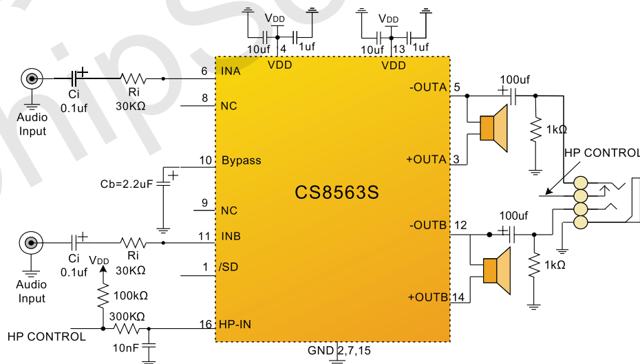
图 1 CS8563S应用线路图
