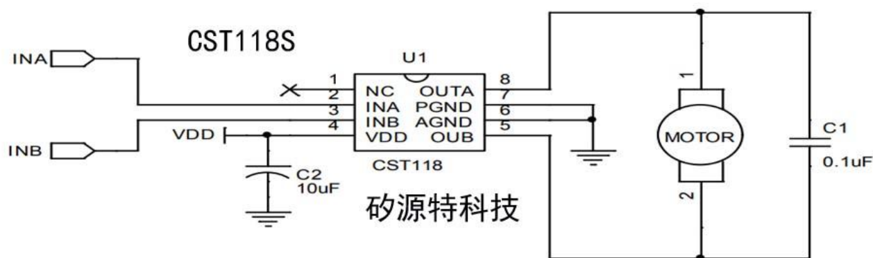
CST118S 低电压低干扰方案应用电路图
