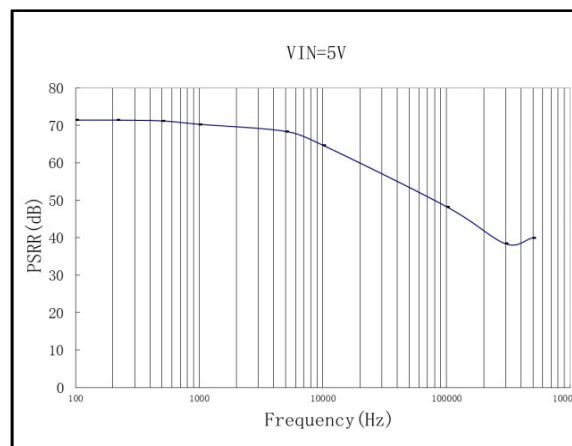
6、PSRR
