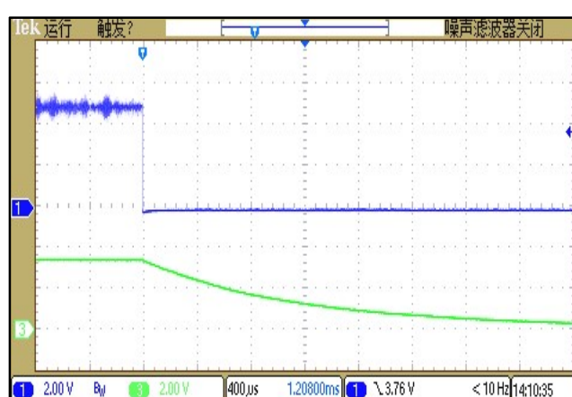
12、Disable
