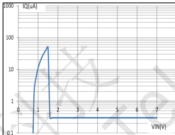
2、IQ vs VIN (※)
