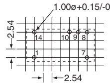
CTDD2010DF-DU3K-1 Footprint
