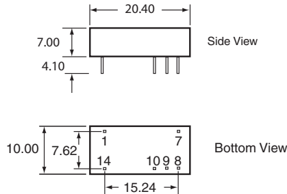
CTDD2010DF-DU3K-1 Footprint
