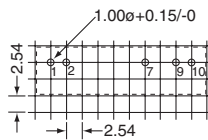
CTDD2709SF-D1K-1 Footprint
