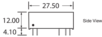
CTDD2709SF-D1K-1 Package
