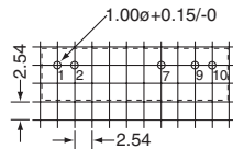
CTDD2710SF-D1K-2 Footprint
