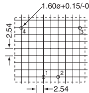
CTDD2727DF-S Footprint
