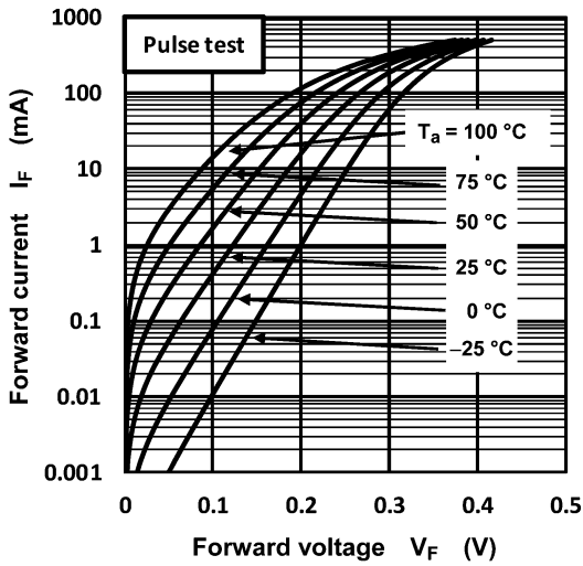
Fig. 8.1 I_F - V_F
