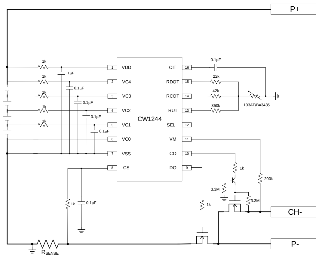
4 串不带均衡功能异口应用电路
