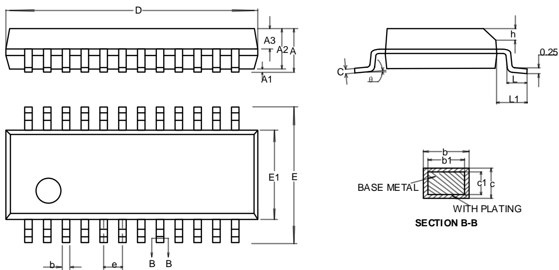
SSOP24 封装
